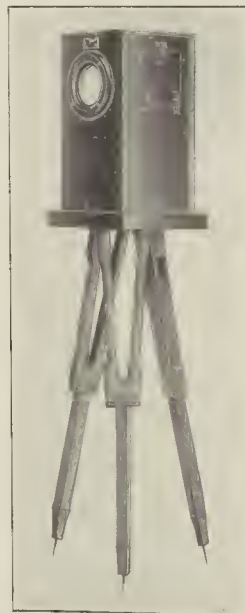
Fig. 2. - El descubridor automático de aguas subterráneas, invento de los Sres. Mansfield y C.º, de Liverpool.
